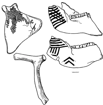
Joonis 22. Mezinist leitud paleoliitilised muusikariistad (Masson 1996: 57).
