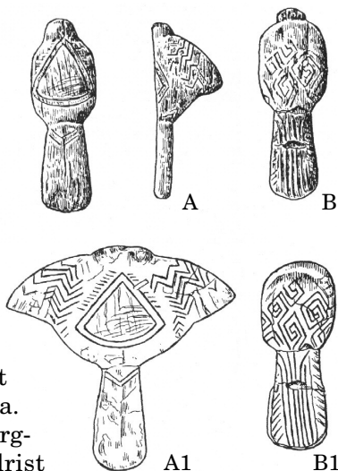
Joonis 19. Mezini linnulaadsed taiesed A ja B ning nende pinnalao- tused A1 ja B1 (Abramova 1962: XXXI).
