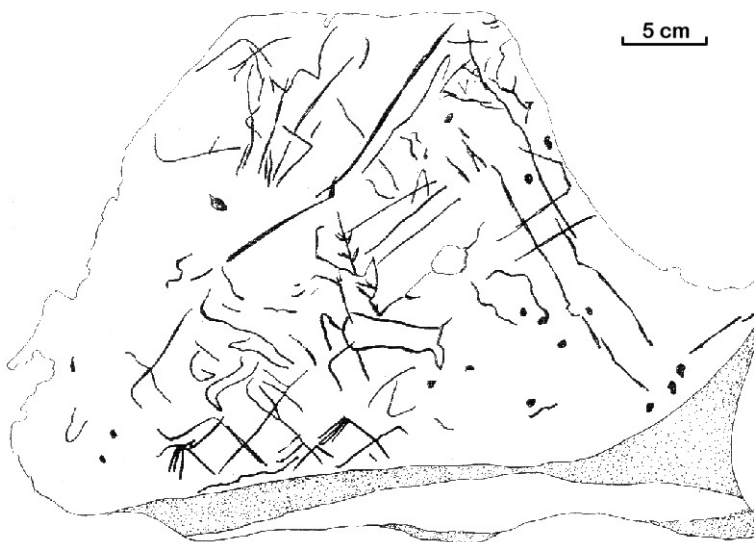
Joonis 14. Enam kui 40 aastatuhande vanune graveering mammuti abaluukatkel (Tšernõš 1978: 22).
