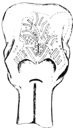
Joonis 17. Punase värviga illustreeritud mammutikolp Mežiritšist (Pidoplitško järgi, Jelinek 1982: 284).
