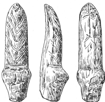
Joonis 20. Mezini falliline taies (Abramova 1962: XXXII).
