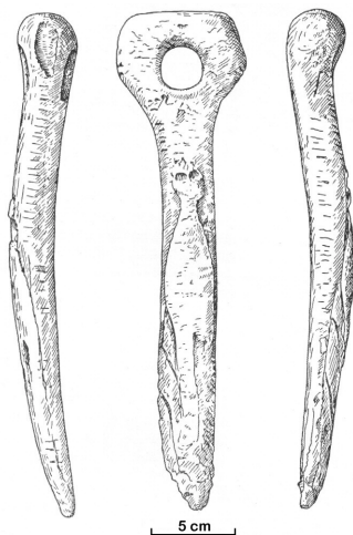
Joonis 16. Madalreljeefse inimlaadse kujutisega sau (Abramova 1962: XL, 5).
